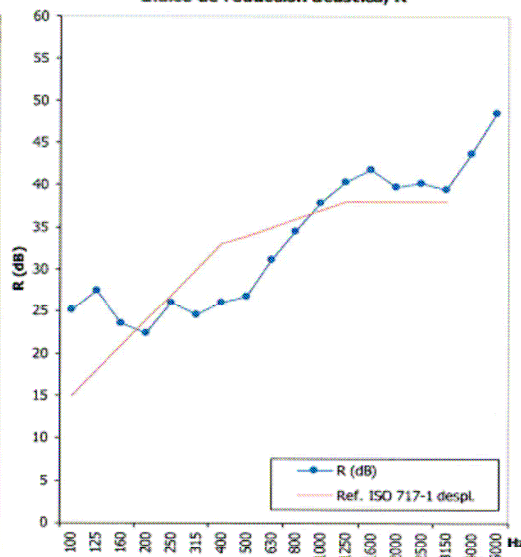
Índice de reducción acústica, R
