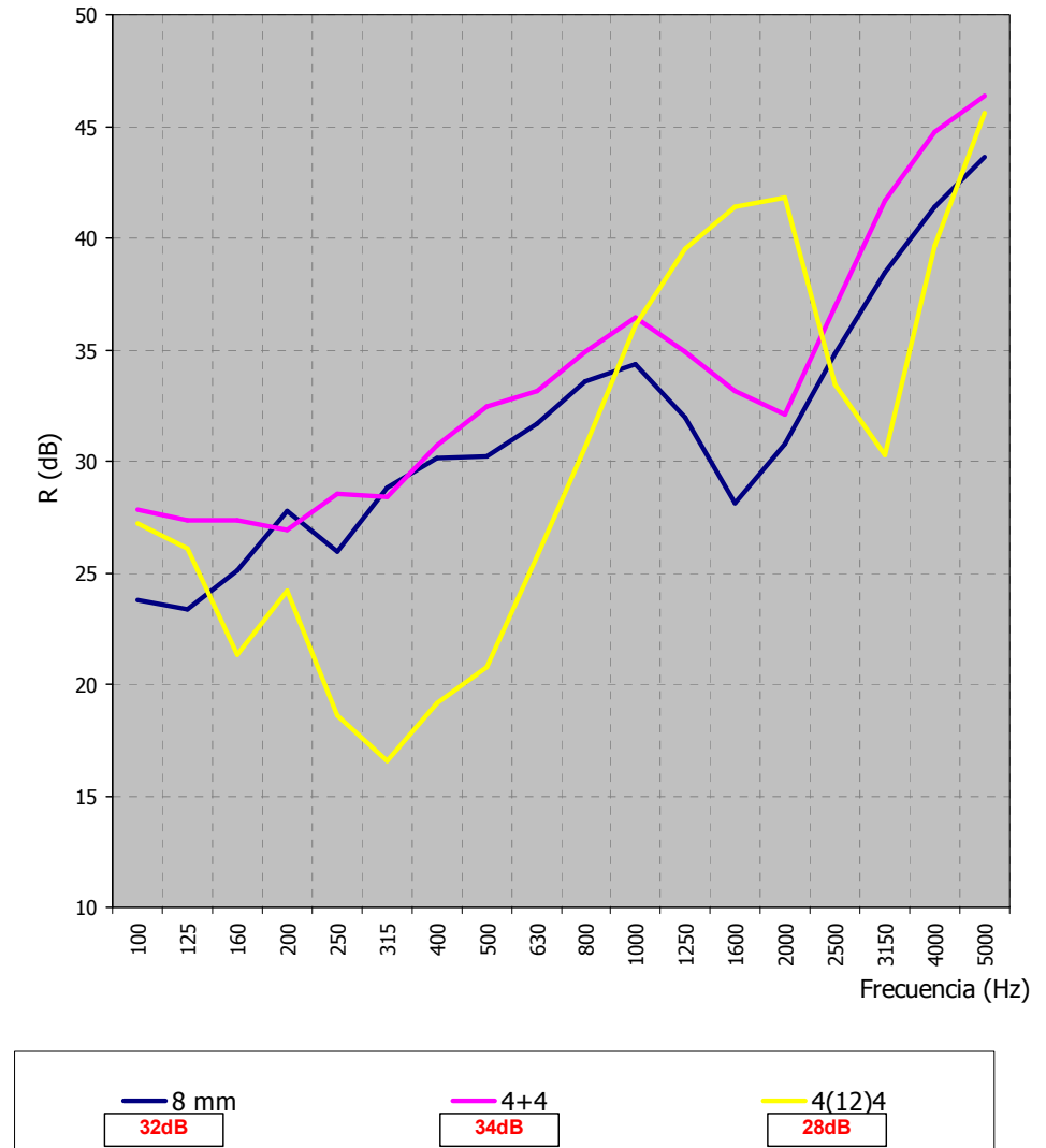
Índice de reducción acústica, R
